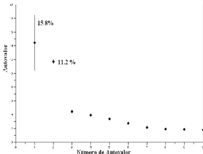
Figura 1: Gráfico “scree” para determinar el número de componentes a usar. En esta figura se muestran los primeros diez autovalores de 146 estaciones de datos diarios localizadas en Mesoamérica (1971 – 2000). Nótese que al haber un traslape de los dos primeros modos se deberían usar ambos para el rellenado de los datos.
